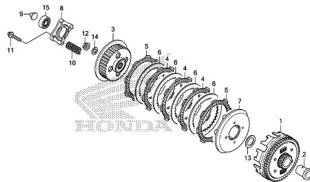
CLUTCH
